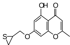
PC-6319101, DMSO-d 6
